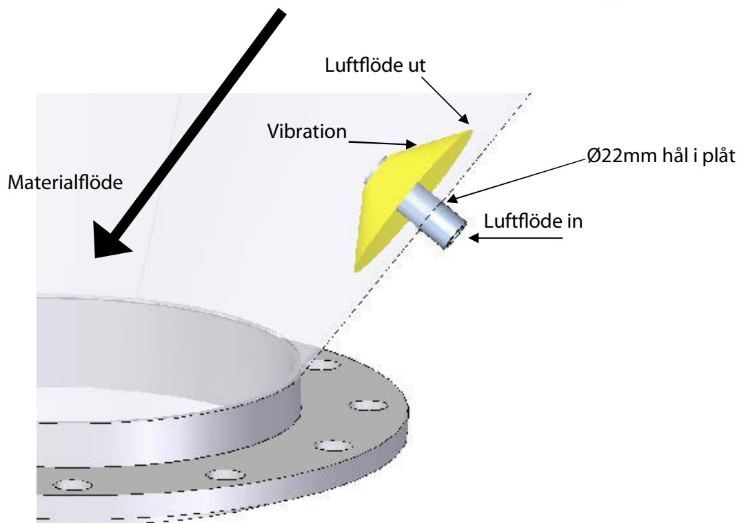
Fluidpad monterad i behållare
