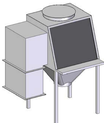
Ensäckstömmaren med komprimatorschakt
